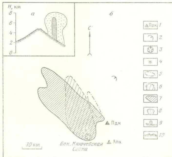
Рис. 4. Изображение на экране локатора вертикального (а) и горизонтальных (б) сечений облака фреатического взрыва в Крестовском желобе Ключевского вулкана 2 декабря 1985 г. 1 — сеймостанция; 2 — локатор; 3 — вершина в. Ключевской; 4 — эпицентр взрыва; 5—7 сечения облака взрыва при углах возвышения антенны локатора 16,7°, 10° и 6,5° соответственно; 8, 9 — периферийная и центральная части облака взрыва; 10 — Ключевской вулкан
