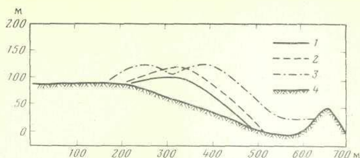
Рис. 5. Профиль шлакового конуса и кромки кратера Ключевского вулкана по линии восток—запад, по данным тригонометрического нивелирования из г. Ключи. Наблюдения выполнены: 1 — 5.II.1984; 2 — 18.III.1985; 3 — 16.V.1986; 4 — кромка кратера
