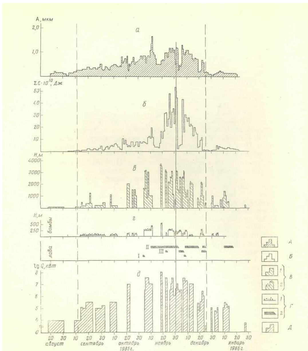
Рис. 2. Характеристики вершинного извержения Ключевского вулкана от 18 августа 1985 г. до 21 января 1986 г. a — ход средней амплитуды вулканического дрожания (ВД), по данным с/ст Апахончич; б — изменение энергии ВД во время извержения; в — изменение высоты парогазовых (1) и газопепловых (2) выбросов во время извержения; г — изменение высоты выбросов вулканических бомб (1) и продолжительность излияния лавовых потоков (2) по Козыревскому [I], Крестовскому [II] и Апахончичскому [III] желобам; д — изменение тепловой мощности эруптивных выбросов во время извержения
