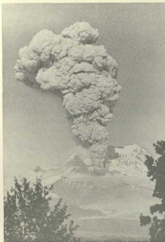
Рис. 1. Газопепловый выброс на вулкане Шивелуч 19 сентября 1985 г. Вид с юга из г. Ключи. Фото А. Ю. Озерова
